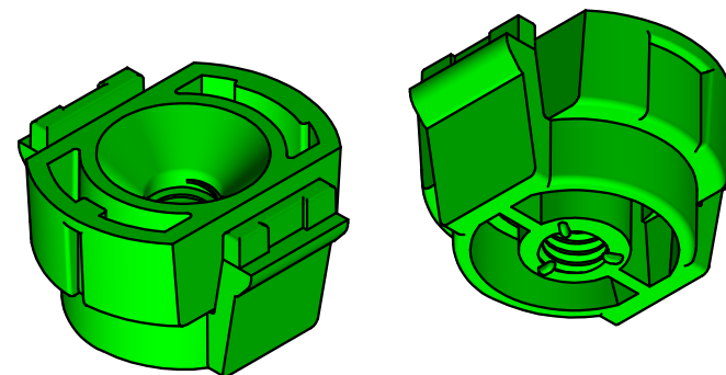
斜視図
