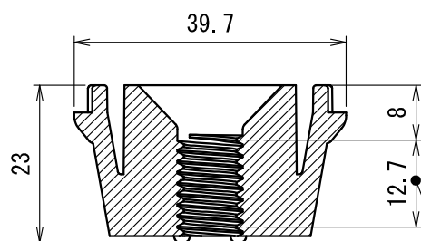
断面 A-A
